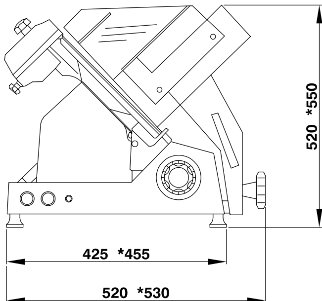
Front aanzicht
