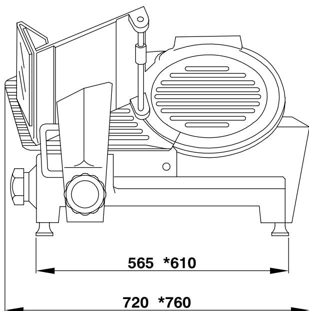
Zij aanzicht
